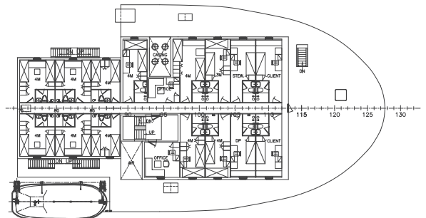
C-deck
