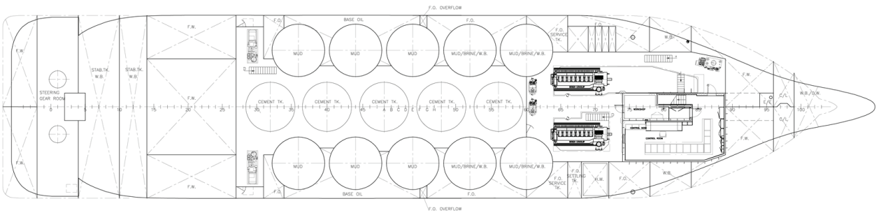
Tween deck
