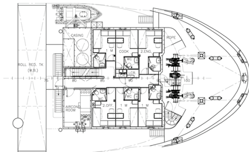
A-deck
